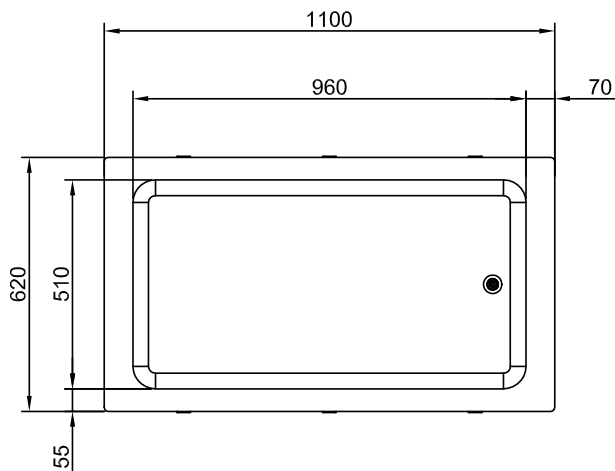
Boven aanzicht
